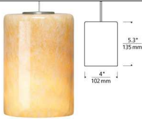
onyx
